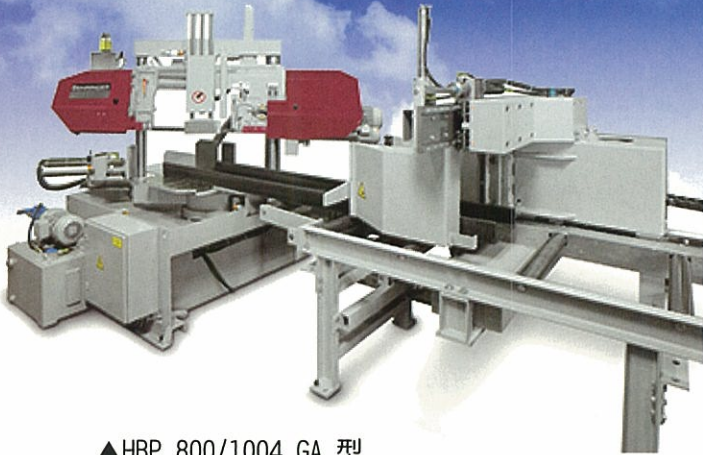
▲HBP 800/1004 GA 型 型材 自動斜切角度定位/定寸帶鋸機 最大工作物規格：棒材 800 mm \phi 型材 (45° 斜切)：590 × 590 mm
