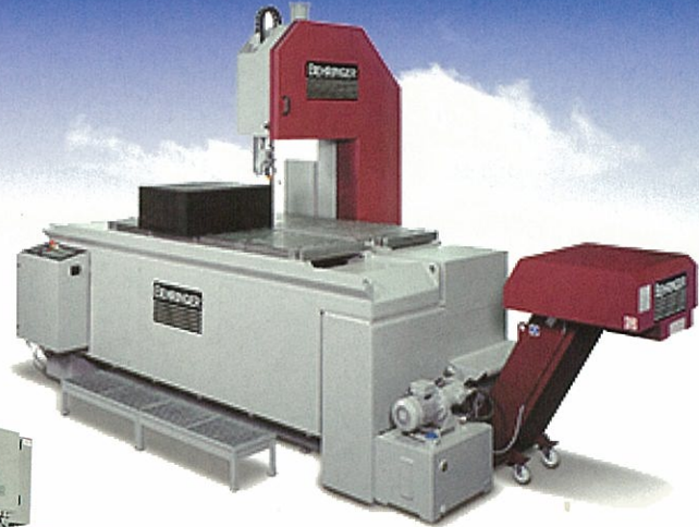
▲LPS 100-120-6 型 方塊鋁/模料 立式裁切帶鋸機 最大工作物規格：長6000 × 寬1200 × 高1000 mm
